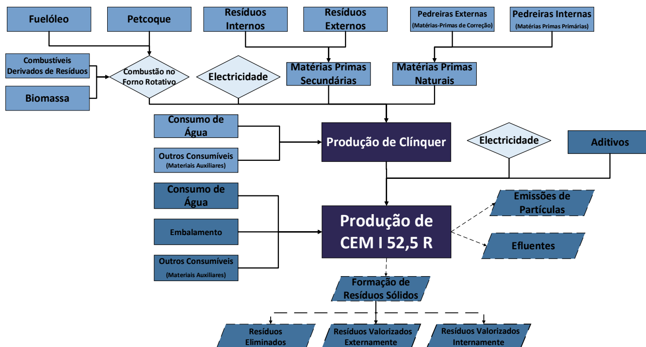
Figura 1: Fluxograma simplificado para o inventário da produção de CEM I 52,5 R.
