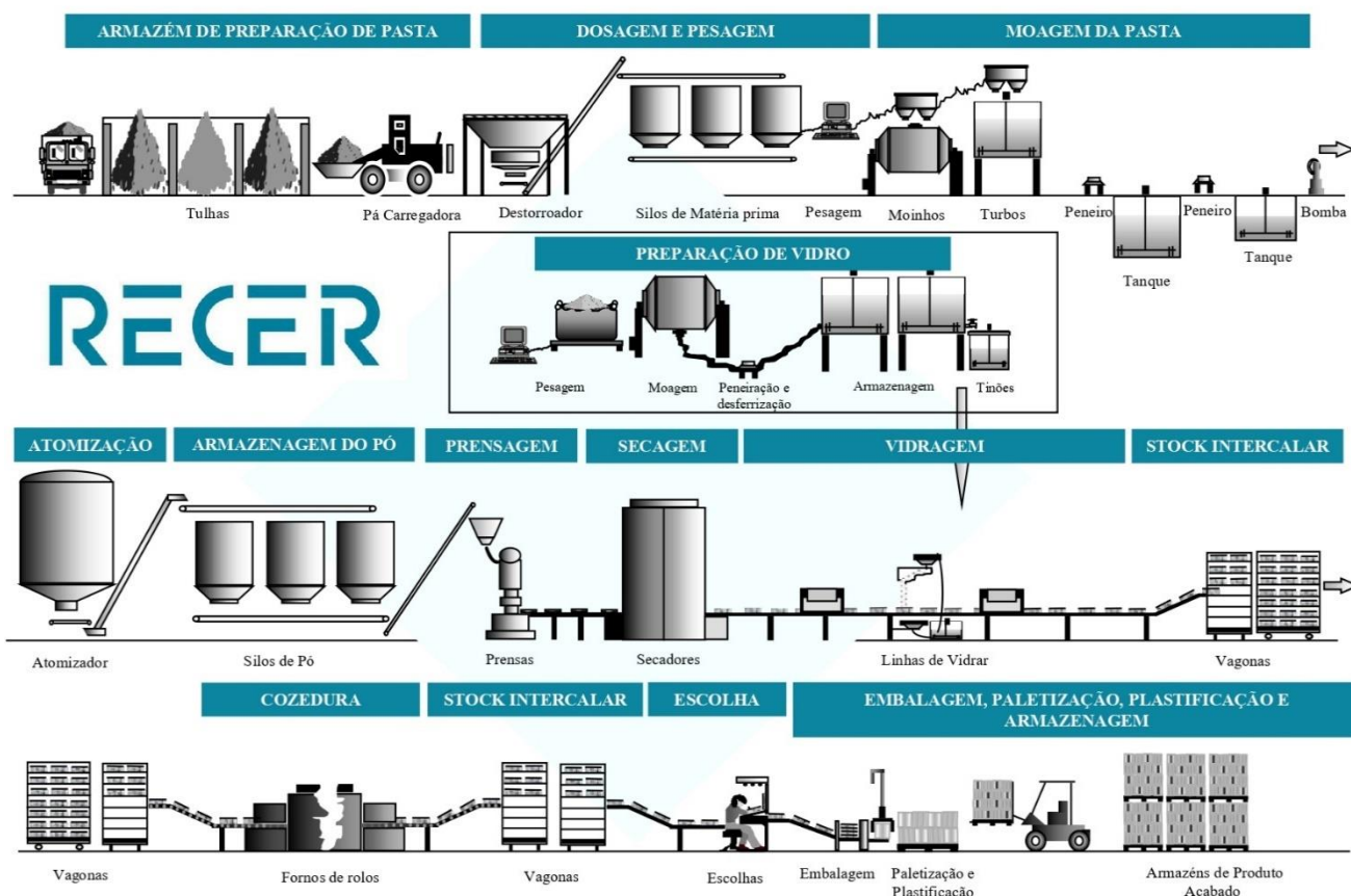
Figura 2 - Processo produtivo
