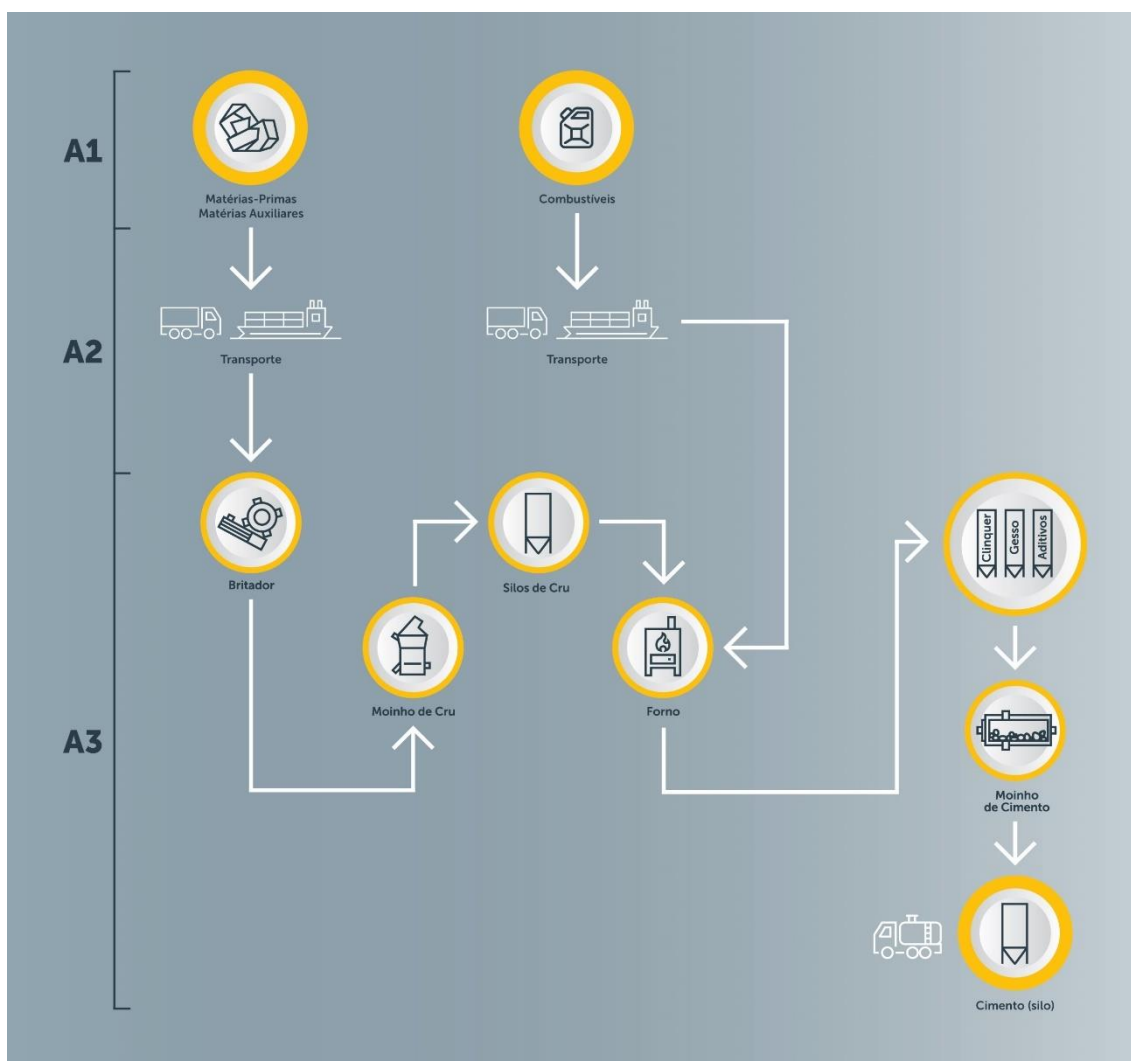
Figura 1: Fluxograma do processo de fabrico do cimento Portland de calcário CEM II/A-L 42,5R
