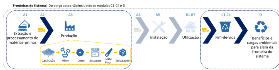
Figura 1: Fronteiras do sistema (do berço ao portão incluindo os módulos C1-C4 e D) da Placa de Gesso Laminado Hidrófuga Gypotec.
