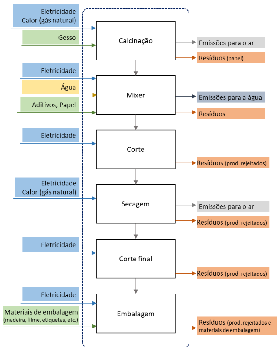
Figura 2: Processo produtivo das placas de gesso laminado Hidrófuga.
