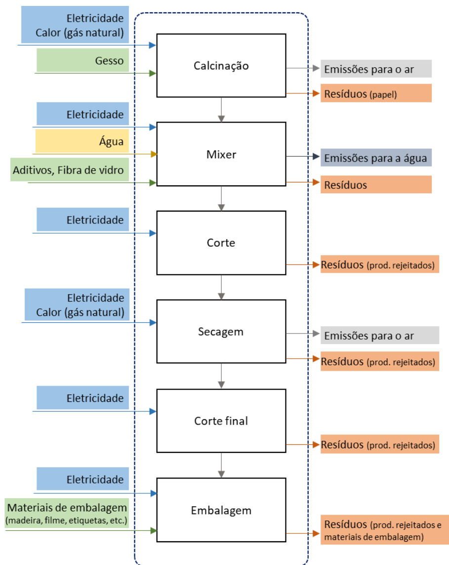
Figura 2: Processo produtivo das placas de gesso laminado Protect.
