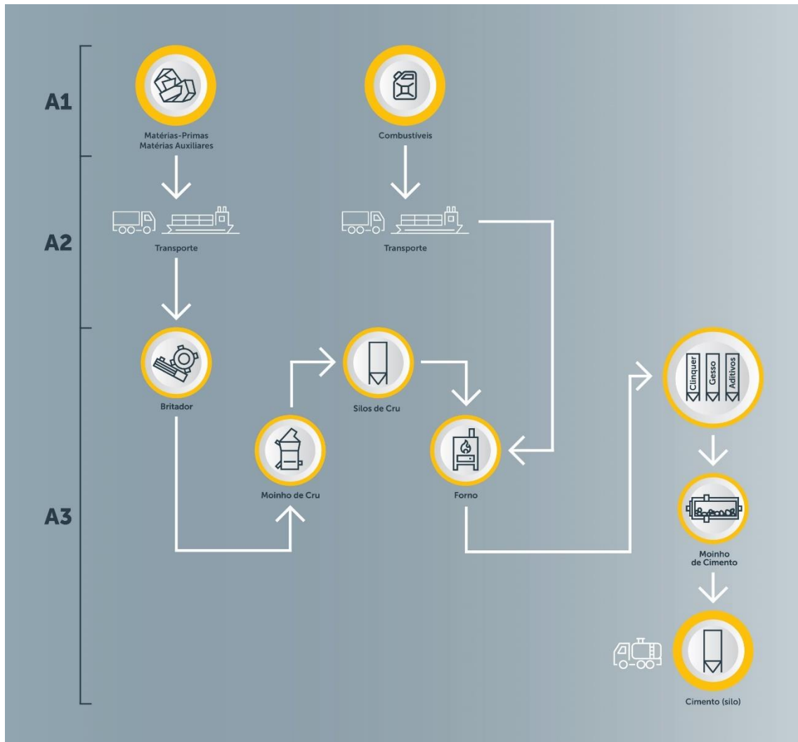
Figura 1: Fluxograma do processo de fabrico do cimento Portland CEM II/B-M (V-L) 42,5R
