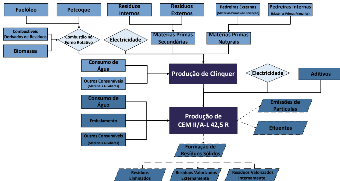
Figura 1: Fluxograma simplificado para o inventário da produção de CEM II/A-L 42,5 R.
