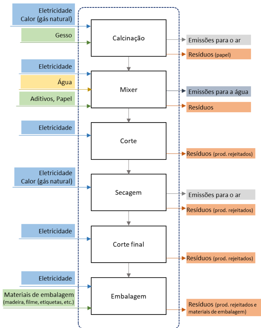
Figura 2: Processo produtivo das placas de gesso laminado Gold.
