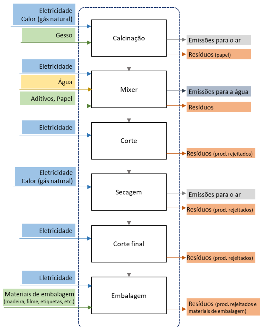
Figura 2: Processo produtivo das placas de gesso laminado Standard.
