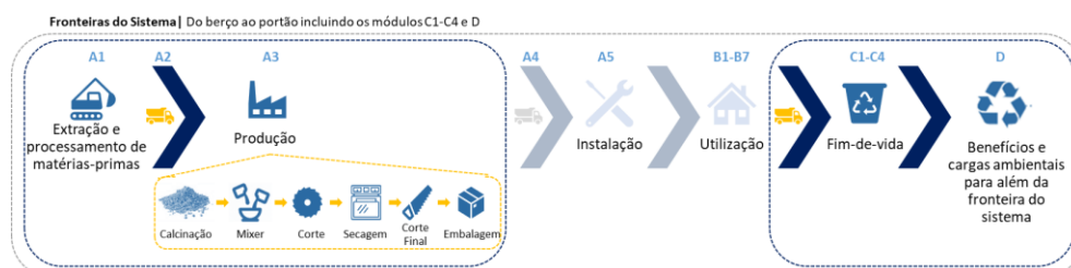
Figura 1: Fronteiras do sistema (do berço ao portão incluindo os módulos C1-C4 e D) da Placa de Gesso Laminado Alta Dureza Gypotec.
