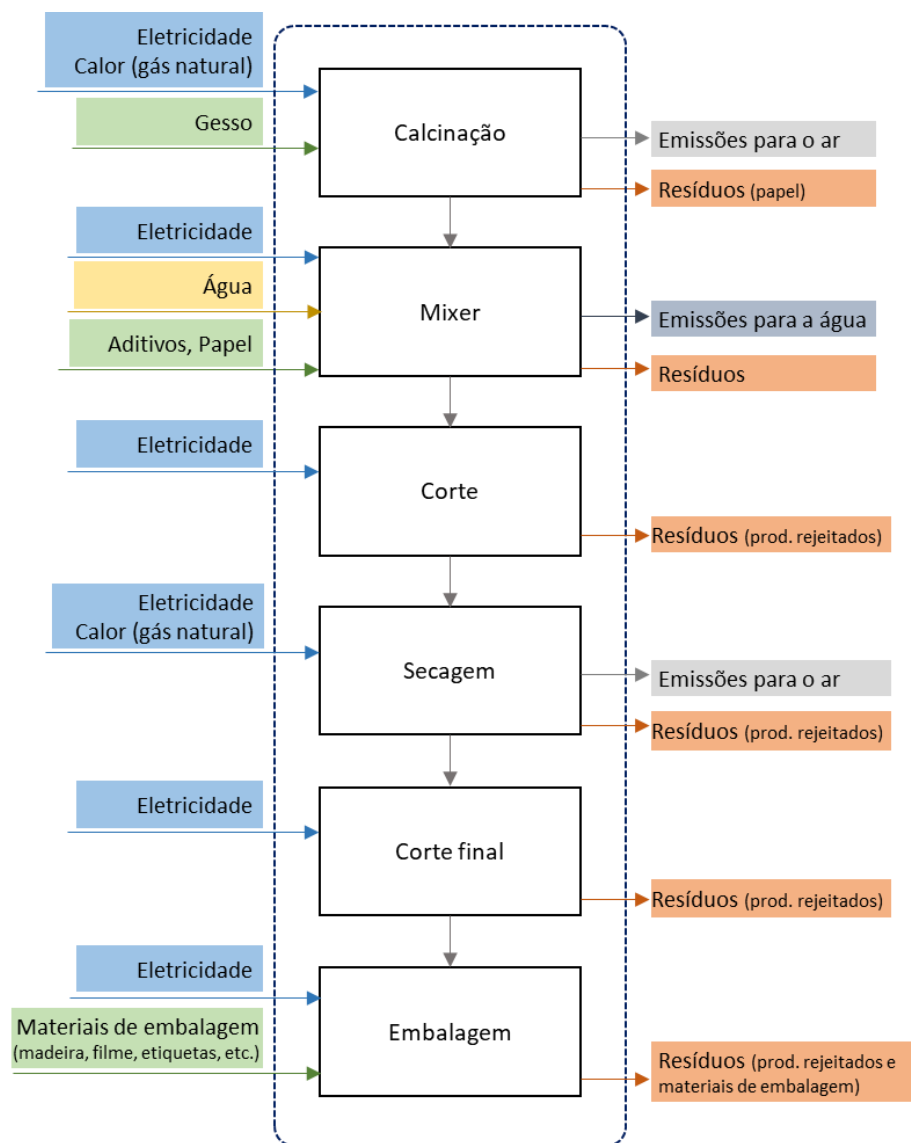
Figura 2: Processo produtivo das placas de gesso laminado Alta Dureza.
