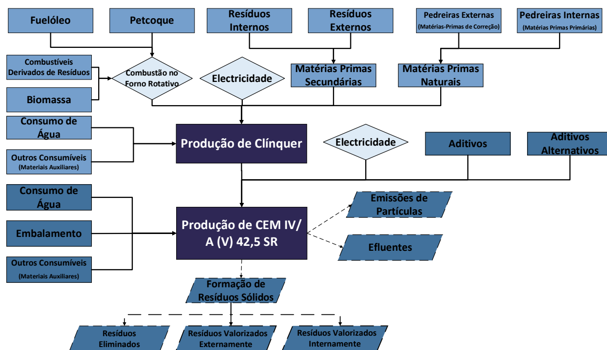
Figura 1: Fluxograma simplificado para o inventário da produção de CEM IV/A (V) 42,5 SR.
