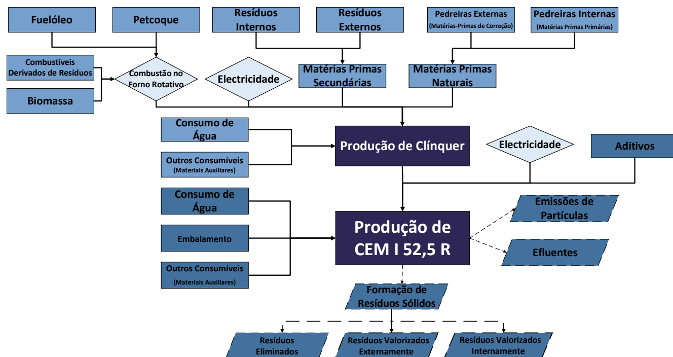
Figura 1: Fluxograma simplificado para o inventário da produção de CEM I 52,5 R.
